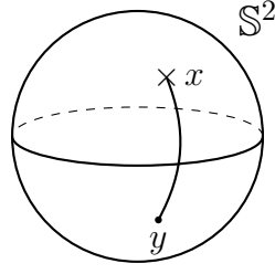
Figura 1: Arco entre x e y en S^2 .
